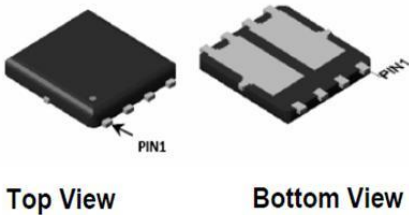
PDFN5x6-8L-D
